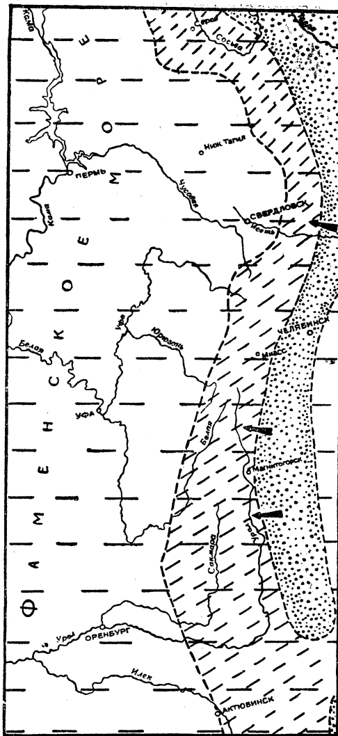
Побережье Фаменского моря, нанесенное на карту палеогеографами. Стрелками показаны наиболее крупные потоки, стекавшие с гористой уральской суши. Полоса вдоль берега — зона песчаных отложений, снесенных с суши.
