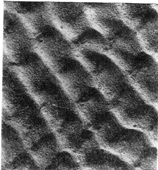
Поверхность пласта песчаника, на которой запечатлены течения двух перекрещивающихся направлений в морском бассейне далекого геологического прошлого.
