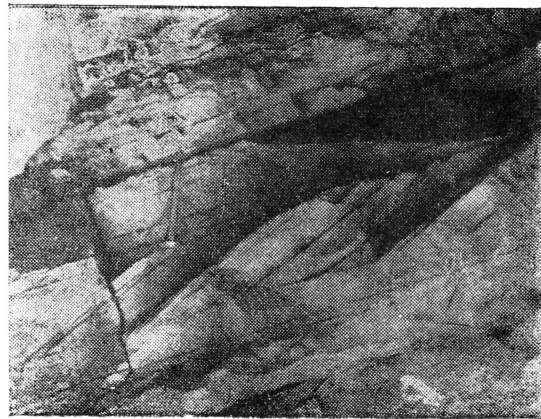
Вот они, косые слои, помогающие палеогеографам определять направление древних потоков.
