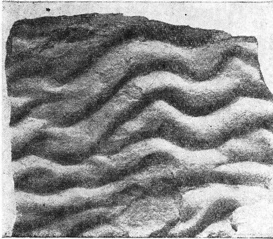
В таком виде на поверхности пласта песчаника сохраняются «следы» воздействия волновых движений древнего моря.
